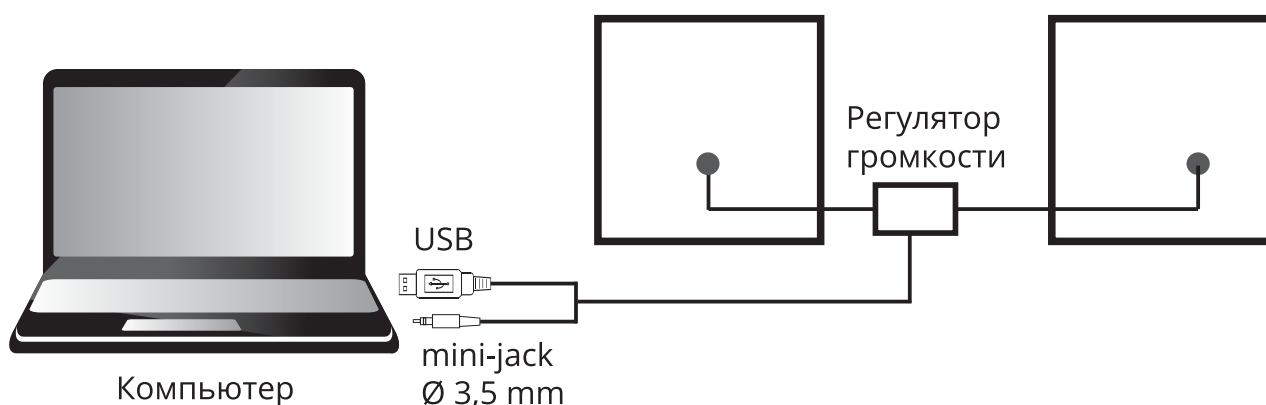
Рис. 1. Схема подключения
